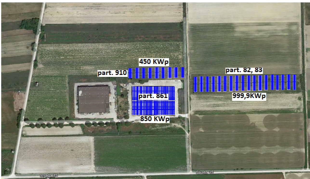
LAYOUT IMPIANTI FOTOVOLTAICI E SUPERFICI INTERESSATE.
