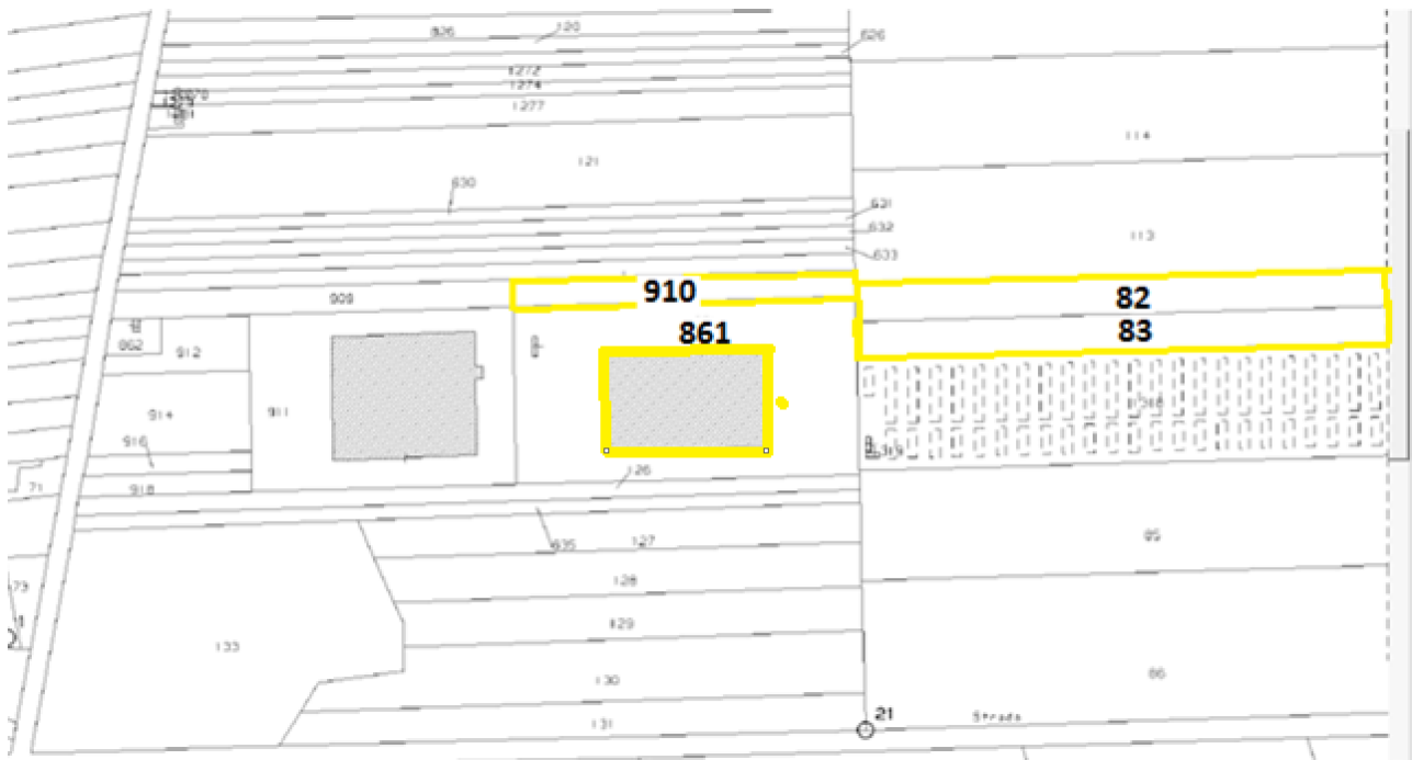
LAYOUT IMPIANTI FOTOVOLTAICI E SUPERFICI INTERESSATE.
